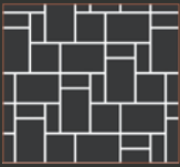
RÖMISCHER VERBAND: 160/80/52 mm 160/160/52 mm 240/160/52 mm
