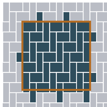
Mailänder Verband
