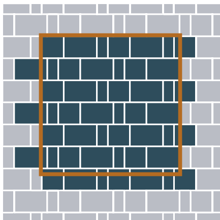
Germanischer Verband
