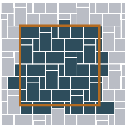
Römischer Verband
